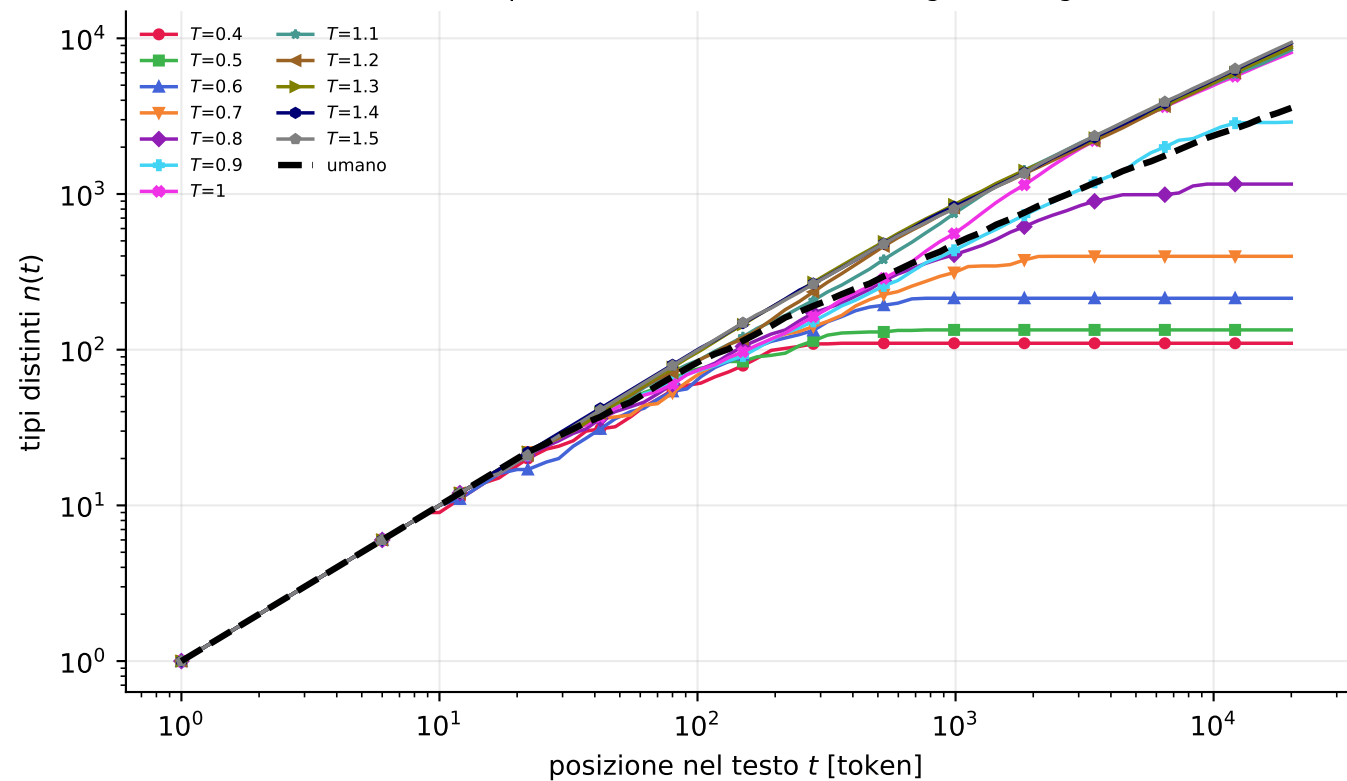
Curve di Heaps — Qwen2.5-1.5B (cfr. [Z] Fig. 3, [L] Fig. 3A)
